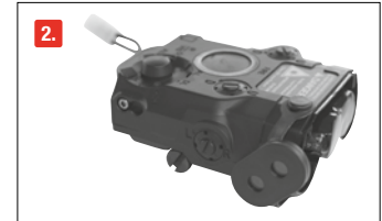
Ouvrez l'obturateur. Introduire la ligne et l'accu comme illustré.
