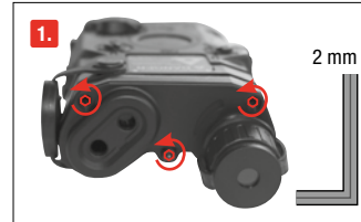
Schrauben lösen
