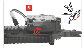
Befestigen Sie die Akkubox auf der Picatinny-Schiene und schließen Sie die Verbindungen an
