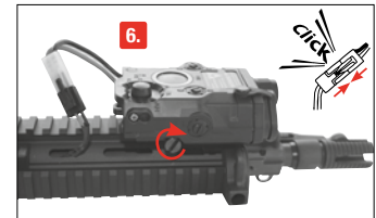
Installez le boîtier de batterie sur le système de fixation par rail, puis connectez les connecteurs
