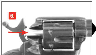
6. Introduire les cartouches dans le barillet.
