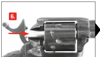
6. Introdurre le cartucce nel tamburo.
